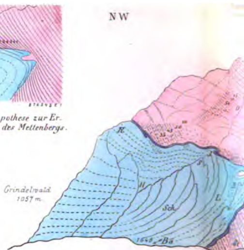
Fig. 4. Der von Gneiss überlagerte Oberjura-Kalkkeil. B - Brunhorn, Ba - Bärgg beim unteren Eismeer, H - Hahnen, L - Langenjahn, O - Obere Jägg, R - Reissen, S - Schneisen, Qt - Eine Quarzbank im Gneiss. Die Zone...
